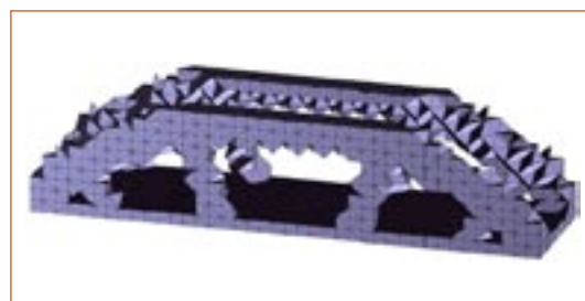
Bild 8: Parameteroptimierung eines Kranauslegers mit “OPIUM”
