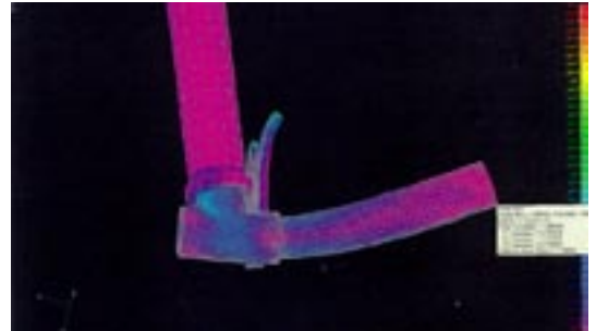
Bild 4: a) Vorderachse mit alten Achsschenkeln aus Stahl b) neuer Achsschenkel aus Aluminium mit Verstellmechanismus und als Hohlwellen ausgeführten Achsen, c) FEM-Analyse
