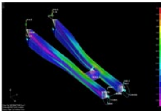
Bild 5: Hinterradschwinge aus Edelstahl: a) Konstruktion, b) FEM-Analyse, c) Fertigung
