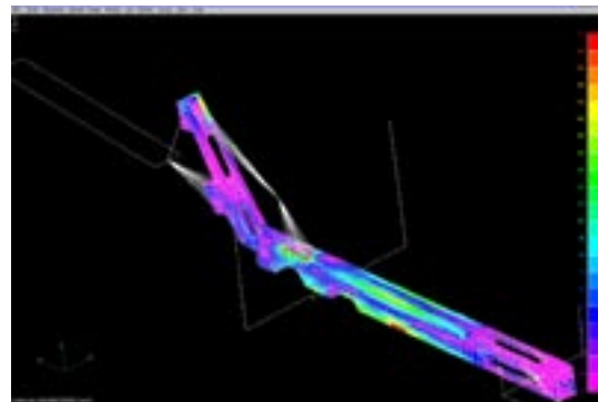
Bild 3: Gewichtsreduzierung des Rahmens: a) Parameteroptimierung der Wandstärke, b) Topologieoptimierung
